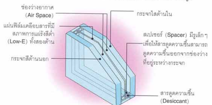
ลักษณะกระจก 2 ชั้นชนิดกันความร้อนเข้าสู่ตัวอาคาร
