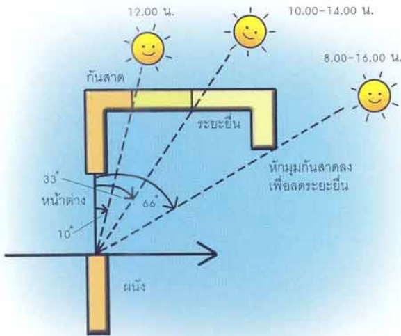
กันสาดทิศเหนือ
